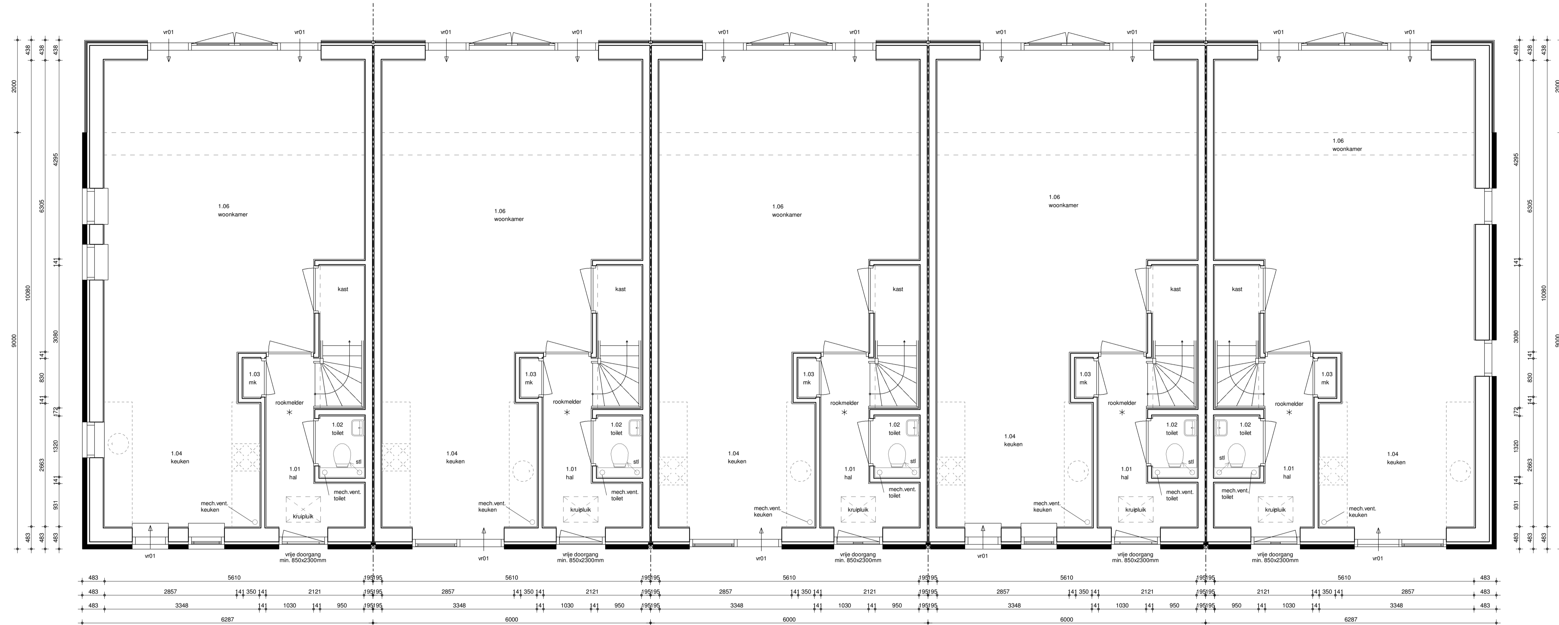
begane grond 1 : 50
