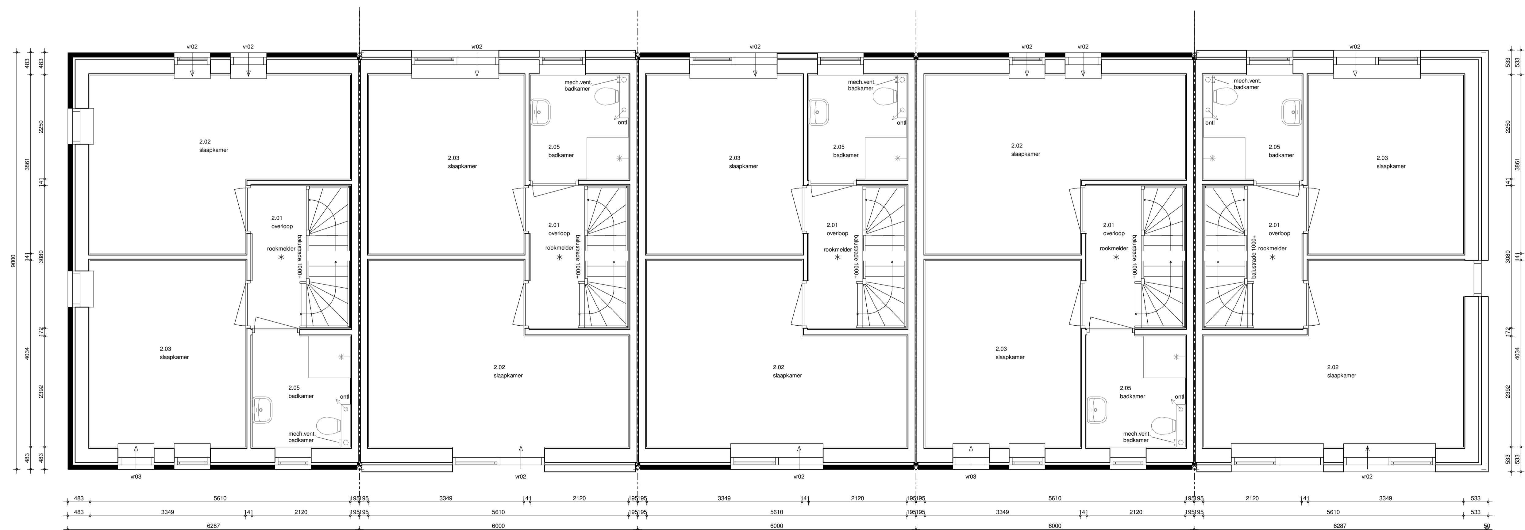
eerste verdieping 1 : 50
